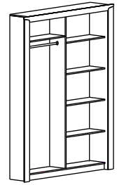
Шкаф-купе 2-х дверный (1380x620x2300)
